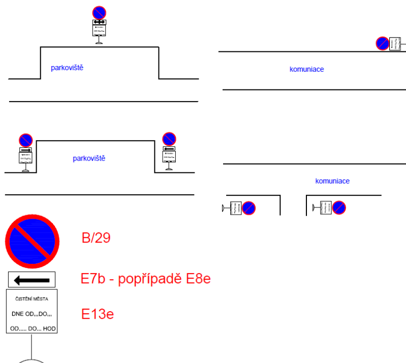
Vzorové umístění přechodného dopravního značení při čištění komunikaci
